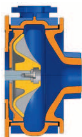
Csésze alakú járókerék profil
