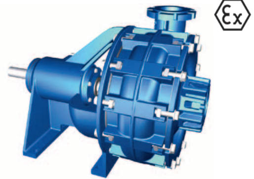
Csupasz tengelyvégű szerelés
