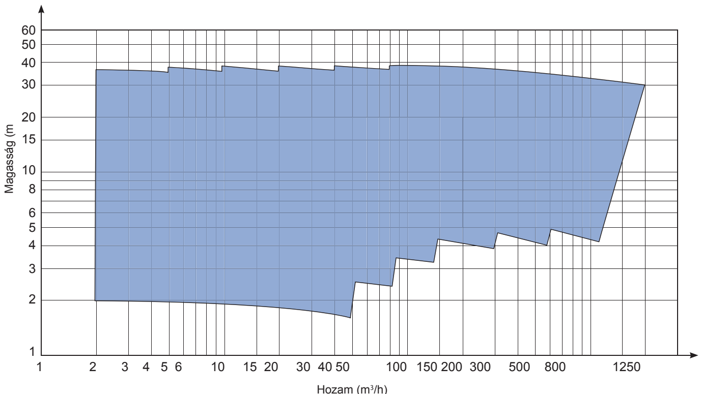
Teljesítmény diagram - Wemco termékcsalád MC. típus - Maximális hozam: 1250 m 3 /h / HMT max : 35 m
