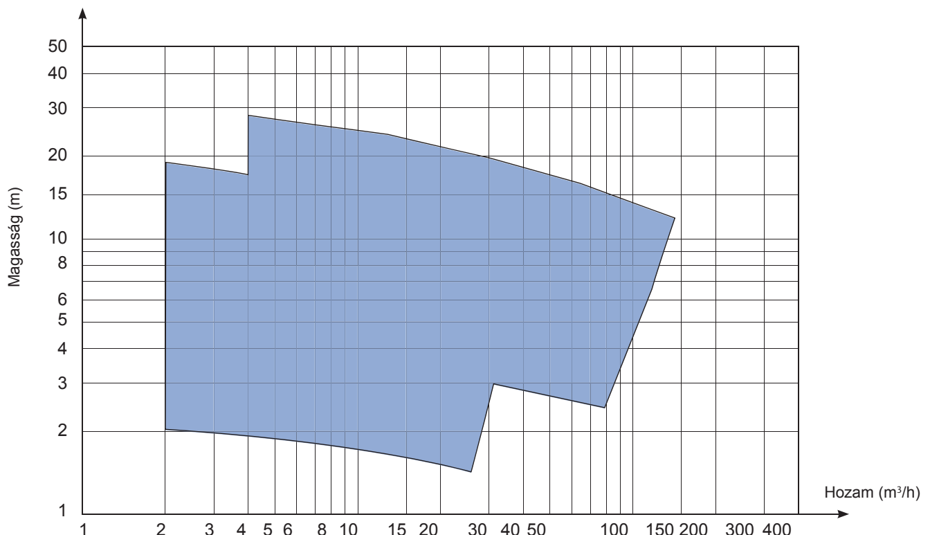
Teljesítmény diagram - Wemco termékcsalád S. típus - Maximális hozam: 150 m 3 /h / maximális emelőmagasság: 30 m
